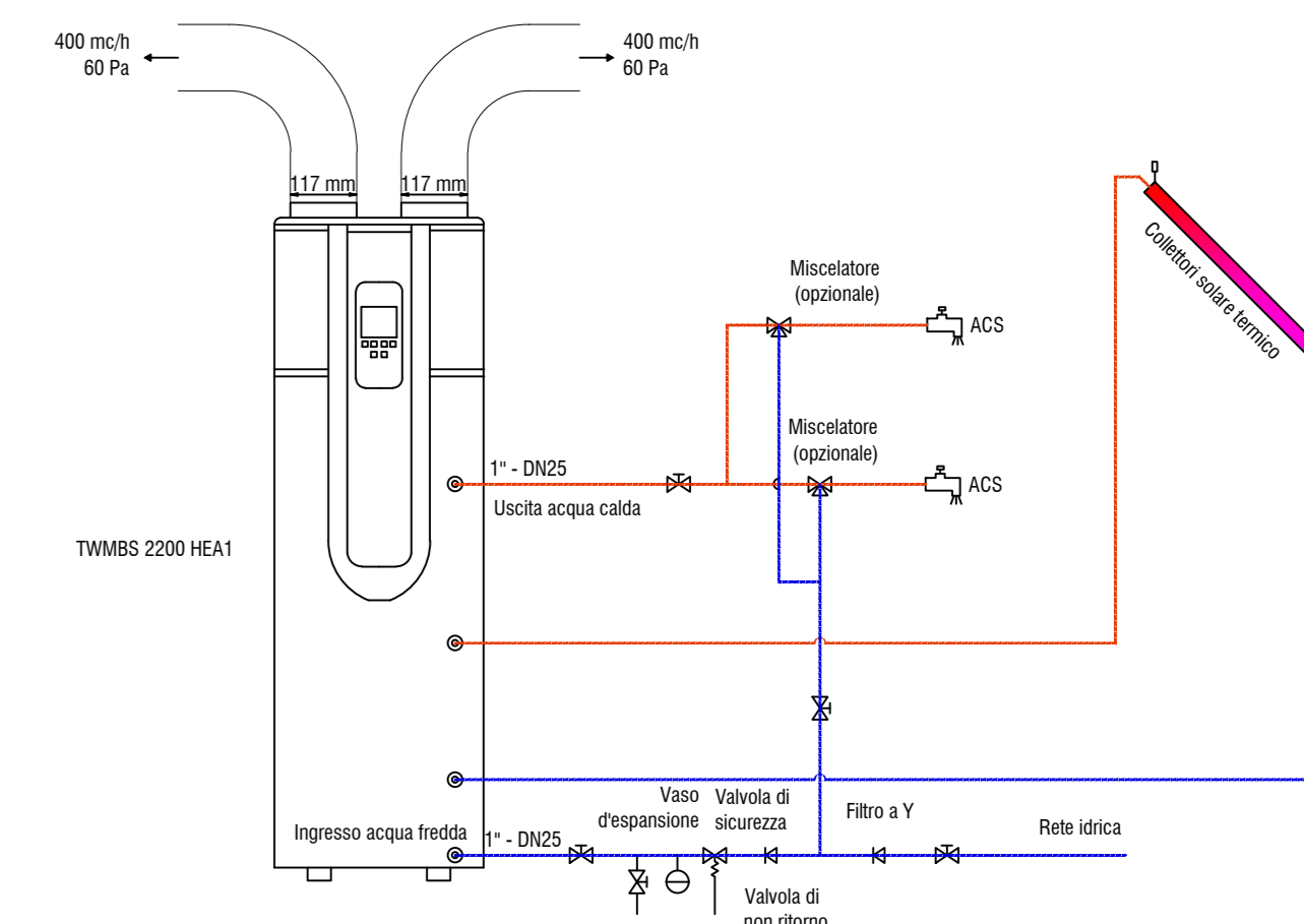
SCHEMA FUNZIONAMENTO HOT WATER
