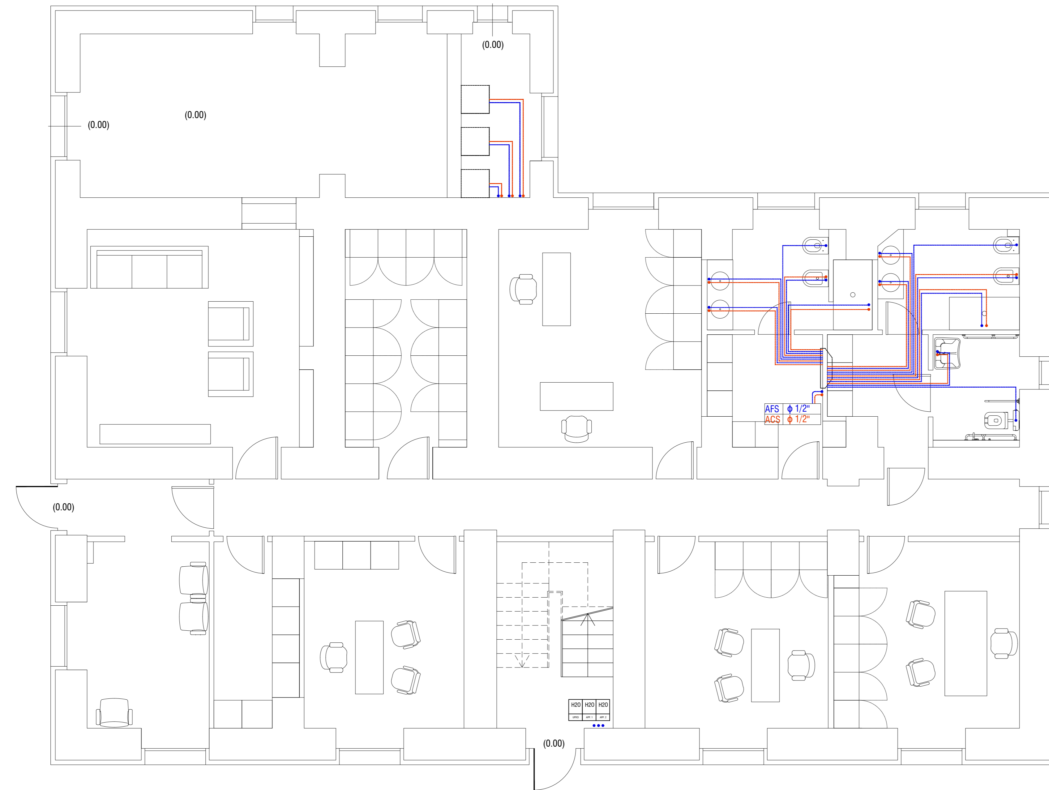
IMPIANTO DI ADDUZIONE ACQUA PIANO TERRA
