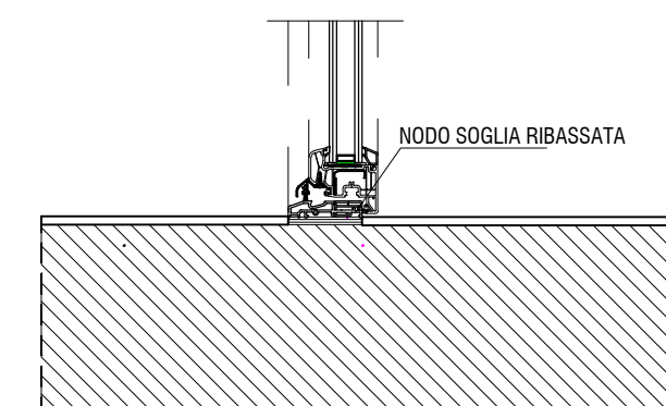
DETAGLIO TELAI INFISSI ESTERNI _ scala 1:10
