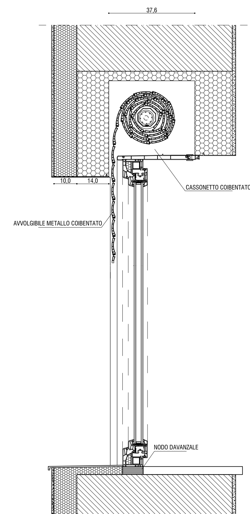
DETAGLIO AVVOLGIBILE _ scala 1:10
