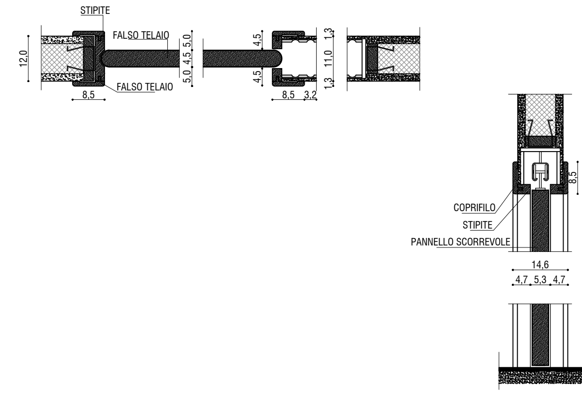
DETAGLIO PORTE INTERNE SCORREVOLI _ scala 1:10
