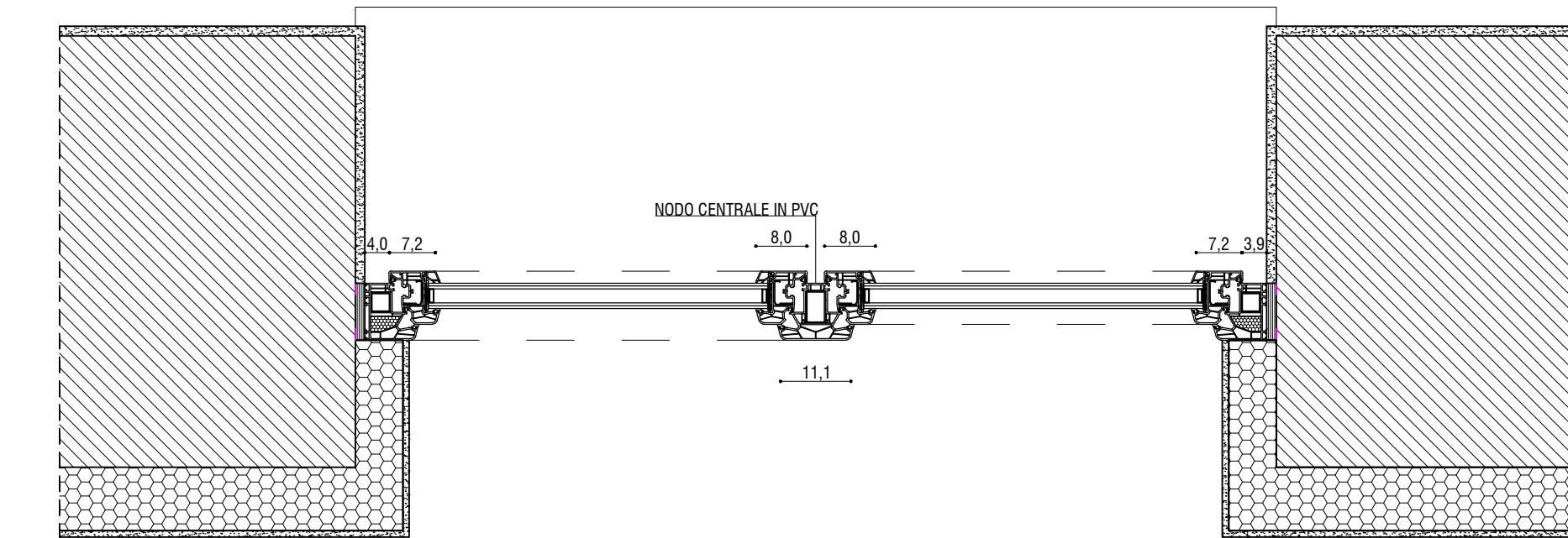
DETAGLIO TELAI INFISSI ESTERNI _ scala 1:10
