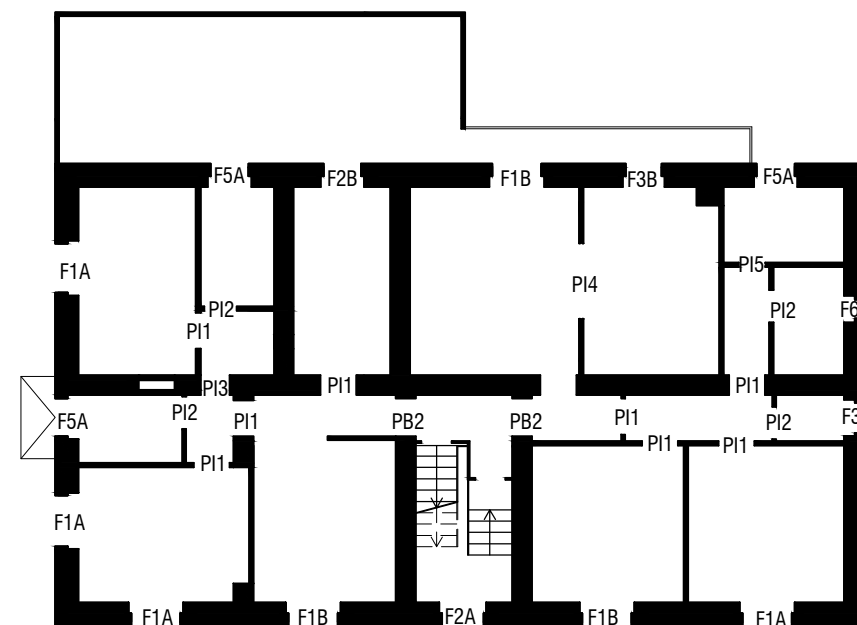
PIANTA PIANO PRIMO _ scala 1:200
