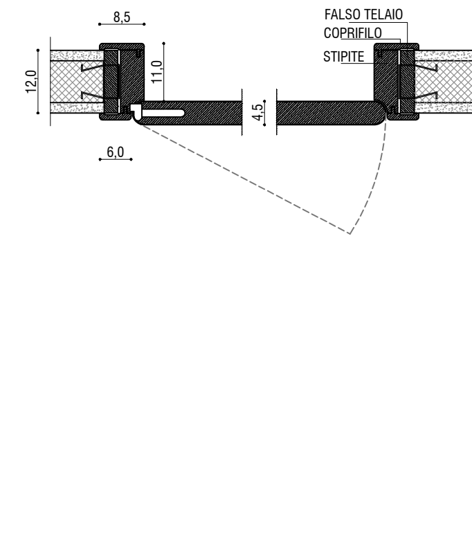
DETAGLIO PORTE INTERNE A BATTENTE _ scala 1:10
